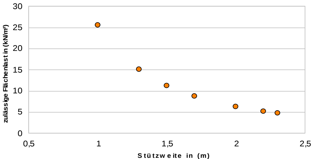
Belastungsdiagramm für systemfreie Rux-Stahlbohlen
