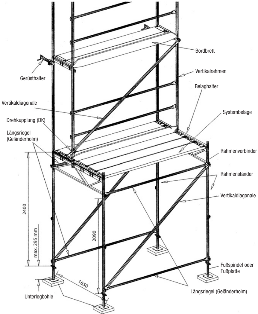
Bild 40 Durchgangsrahmen mit aufgesetztem Vertikalrahmen
