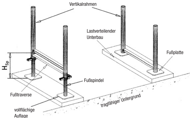
Bild 1a Lastverteilernder Unterbau mit Gerüstbohlen
