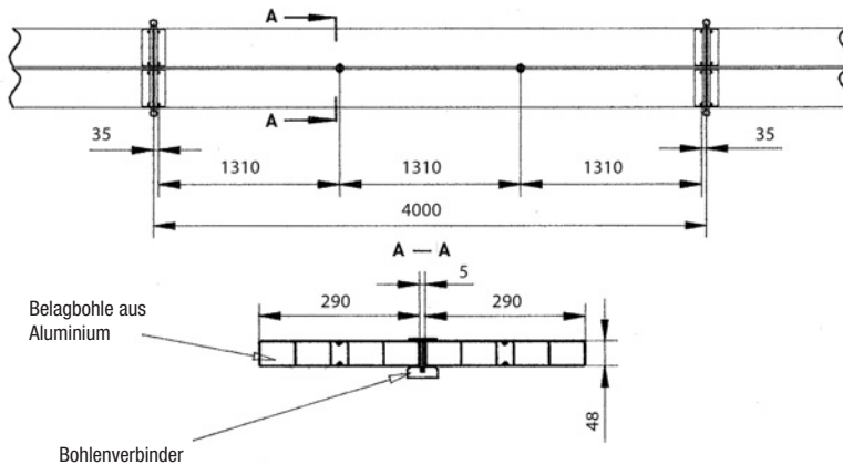
Bild 47 Anordnung der Bohlenverbinder
