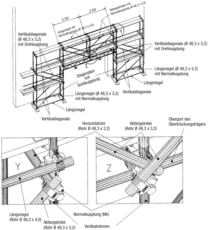
Bild 46a Aufbau mit Abfangstreben; Aussteifung der Obergurtenebene durch Verankerung an der Fassade oder durch Horizontalverband; Gerüstfeldlänge l = 2,50 m
