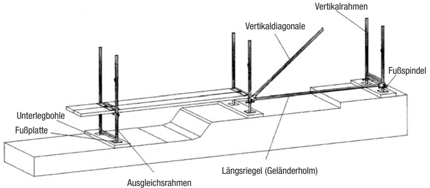
Bild 3 Aufbau mit vertikalem Ausgleichsrahmen
