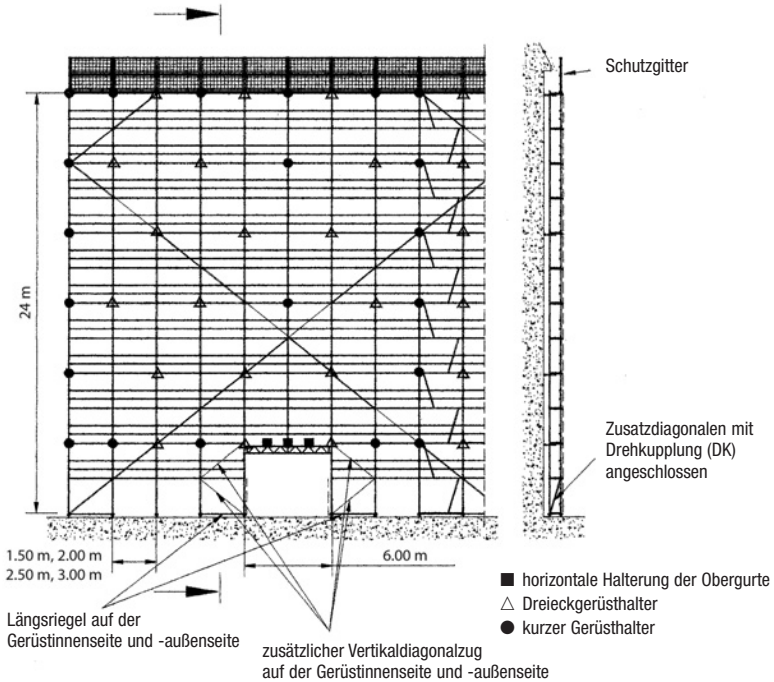
Bild 43b Überbrückungsträger l = 6,00 m eingebaut (ohne Abfangstreben, unbedecktes Gerüst)
