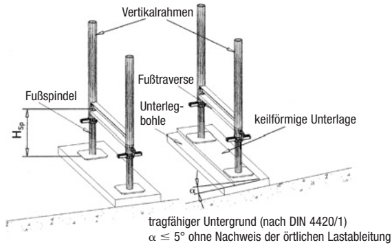
Bild 1b Beispiele für die Auflagerung
