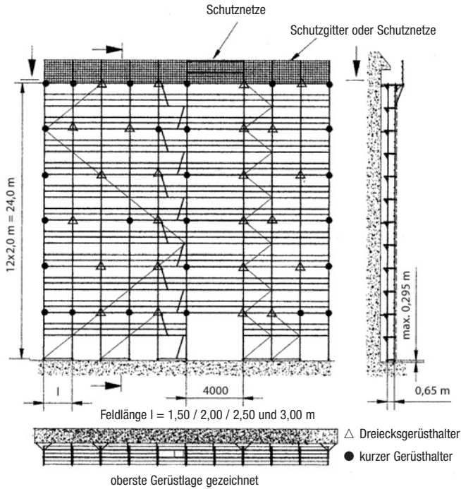
Bild 48 unbedecktes Gerüst vor offener oder geschlossener Fassade mit Überbrückungsfeld l = 4,00 \text{ m} , mit Innen- und Außenkonsolen, mit oder ohne Schutzgitter bzw. -netze
