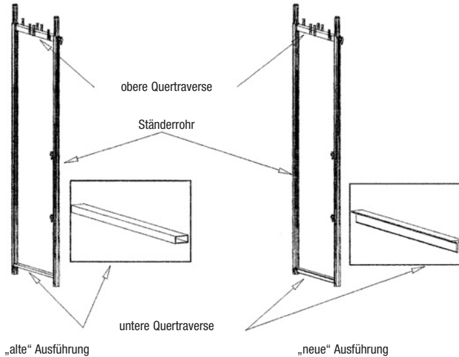
Bild 14 „alte“ und „neue“ Ausführung der Vertikalrahmen
