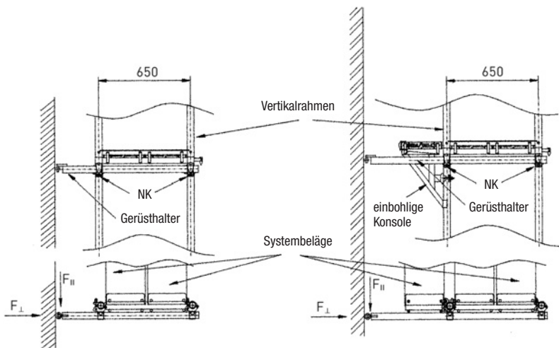
Bild 12 Lange Gerüsthalter
