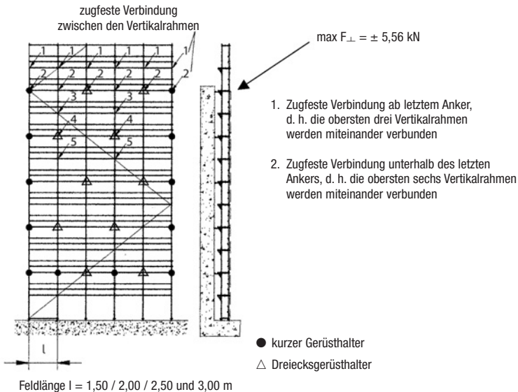
Bild 52 Über der letzten Verankerung freistehende Gerüstlagen; unbekleidetes Gerüst mit Innenkonsolen vor offener Fassade
