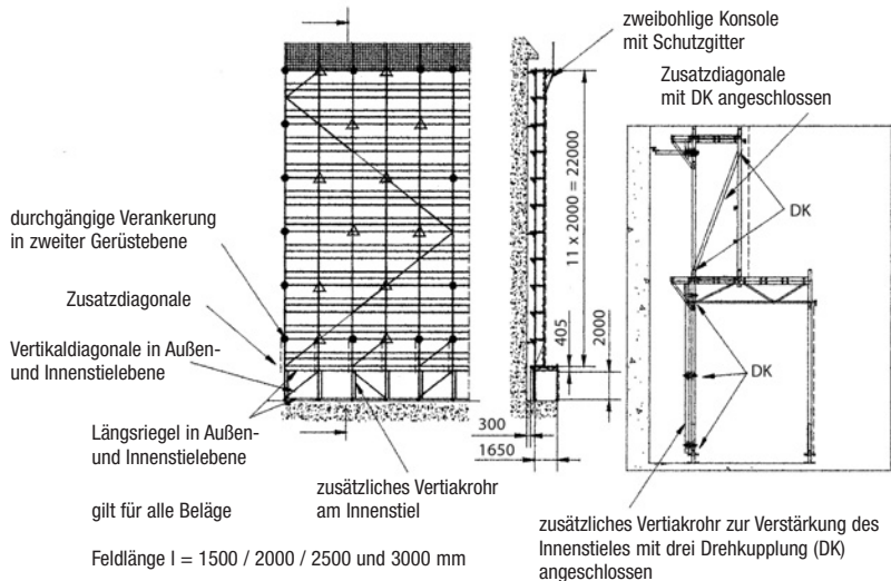
Bild 41c unbekleidetes Gerüst vor offener oder geschlossener Fassade mit Innen- und Außenkonsolen, mit und ohne Schutzgitter
