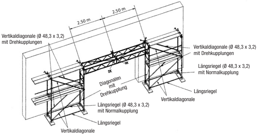
Bild 45a Aussteifung der Obergerurtebene durch Horizontalverband; Gerüstfeldlänge l = 2,50 m (nur für unbedeckte Gerüste)
