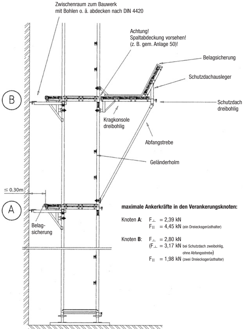
Bild 49 Schutzdachausleger
