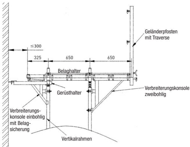
Bild 42 Anordnung von Verbreiterungskonsolen in der obersten Gerüstlage
