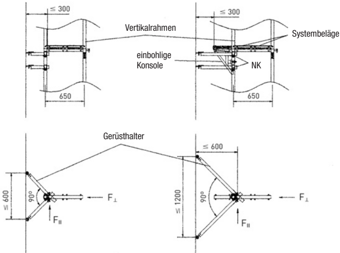
Bild 13 Dreiecksgerüsthalter
