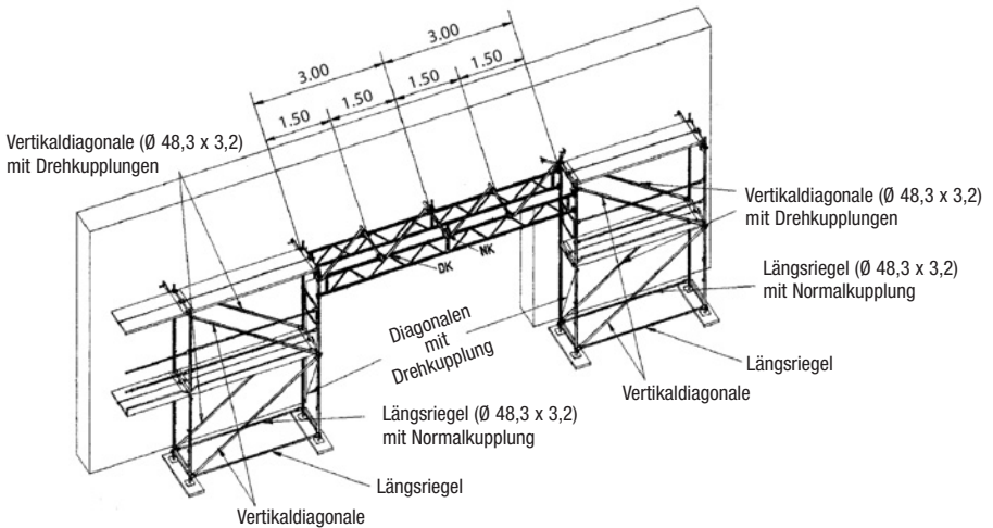
Bild 45b Aussteifung der Obergerurtebene durch Horizontalverband; Gerüstfeldlänge l = 3,00 m (nur für unbedeckte Gerüste)
