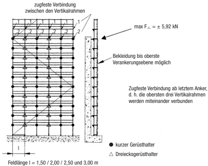
Bild 54 Über der letzten Verankerung freistehende Gerüstlagen; Gerüst mit Planen bekleidet und mit Innenkonsolen
