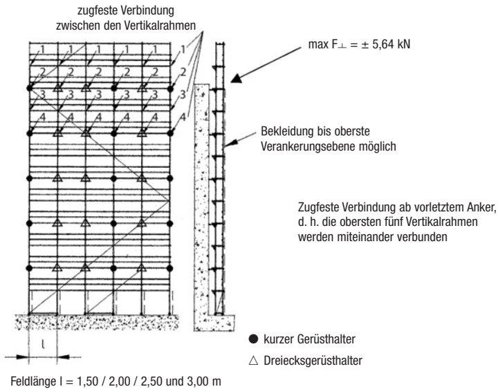
Bild 53 Über der letzten Verankerung freistehende Gerüstlagen; Gerüst mit Netzen bekleidet und mit Innenkonsolen vor offener Fassade
