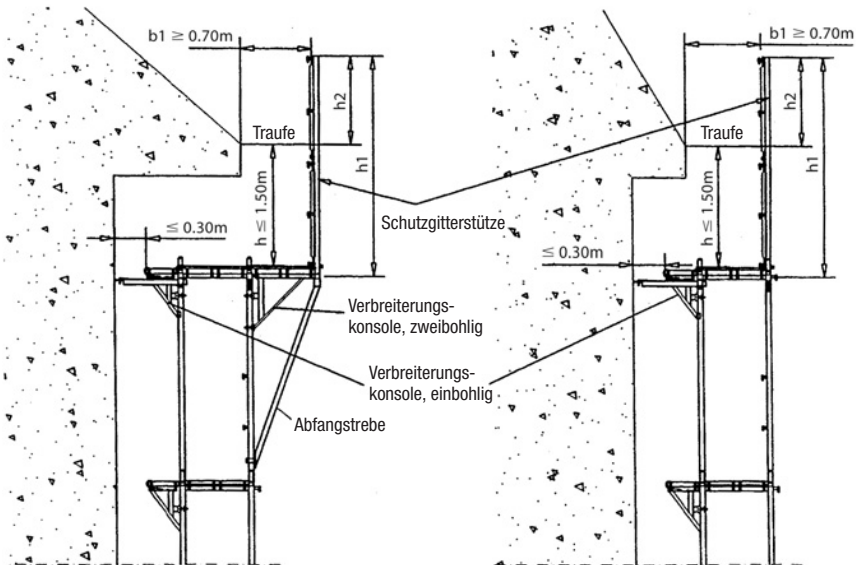
Bild 50 Dachfangerüst
