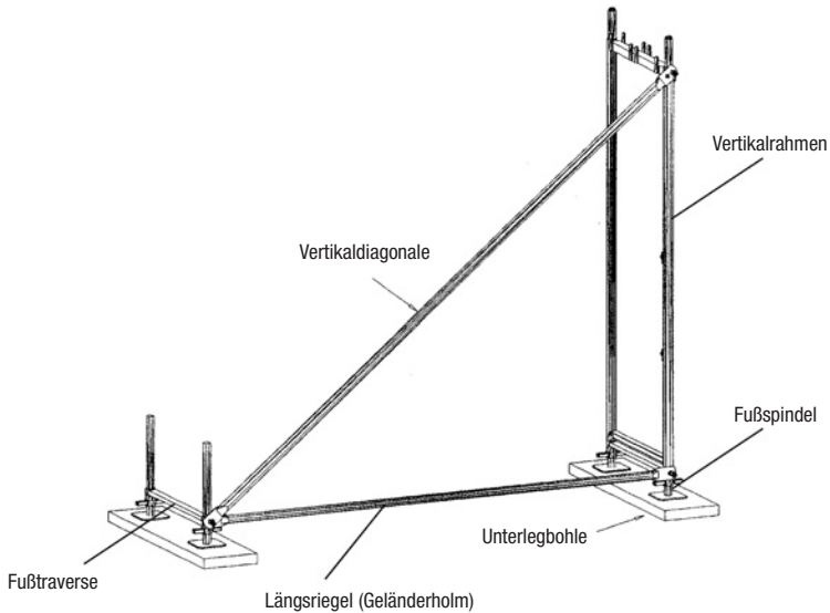
Bild 4 Aufsetzen des Vertikalrahmens und gleichzeitige Standsicherung mittels Vertikaldiagonale
