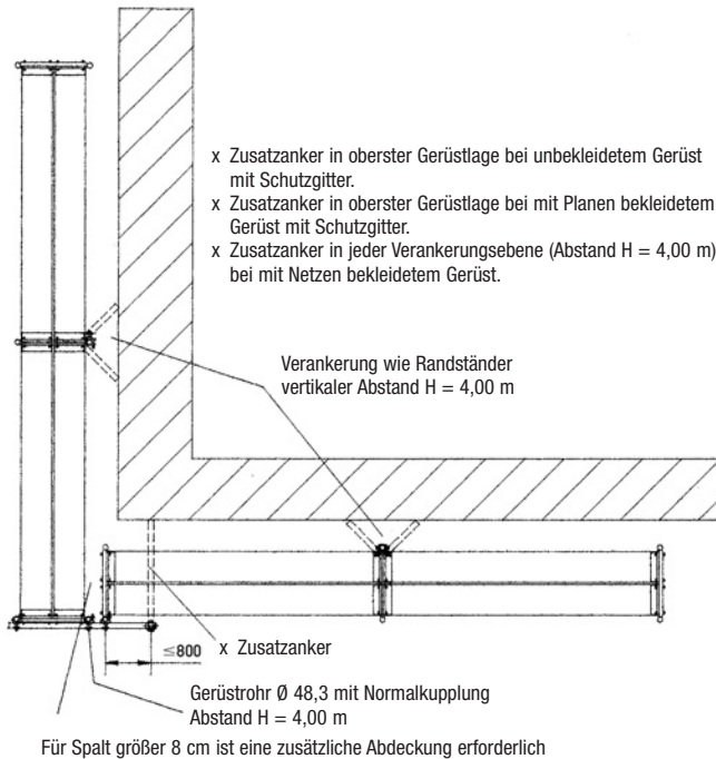
Bild 7a Eckausbildung durch Verbindung der Rahmenständer mittels Gerüstrohr und Normalkupplung. In oberster Gerüstlage ist bei Einsatz eines Schutzgitters ein weiterer Anker im Eckbereich erforderlich
