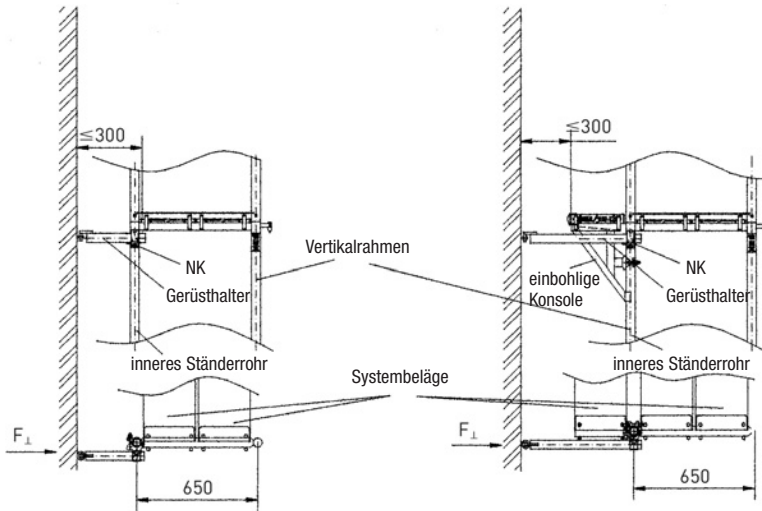
Bild 11 Kurze Gerüsthalter
