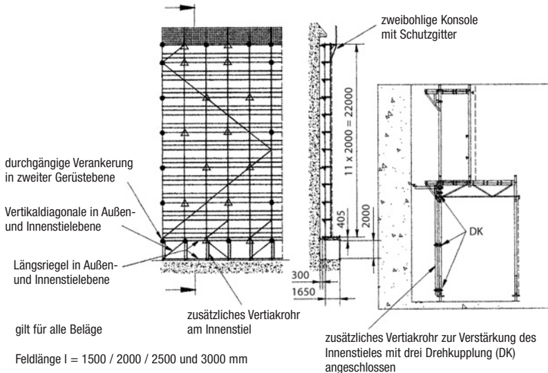
Bild 41e unbekleidetes Gerüst vor offener oder geschlossener Fassade mit Innen- und Außenkonsolen, mit und ohne Schutzgitter
