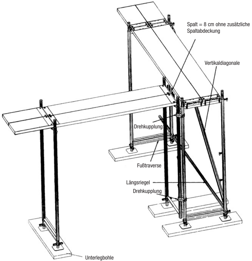
Bild 7b Eckausbildung durch Anschluß mit Drehkupplungen
